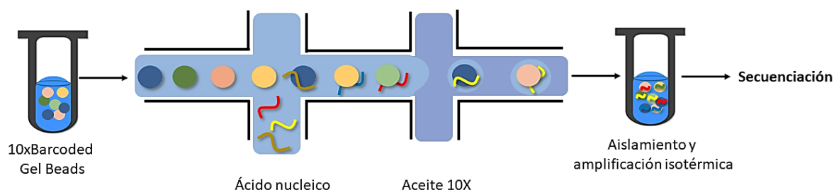
Figura 4: Representación esquemática del funcionamiento de la tecnología basada en microfluídica de 10X Genomics. Las partículas marcadas que contienen todo lo necesario para la amplificación isotérmica pasan al sistema microfluídico donde entran en contacto con fragmentos de ADN de alto peso molecular. Tras la formación del complejo partícula-fragmento, con la ayuda de un aceite altamente concentrado, se procede al aislamiento de los fragmentos de ADN unidos a las partículas y su amplificación isotérmica. Tras la amplificación isotérmica se procede a la secuenciación mediante la plataforma Illumina.
